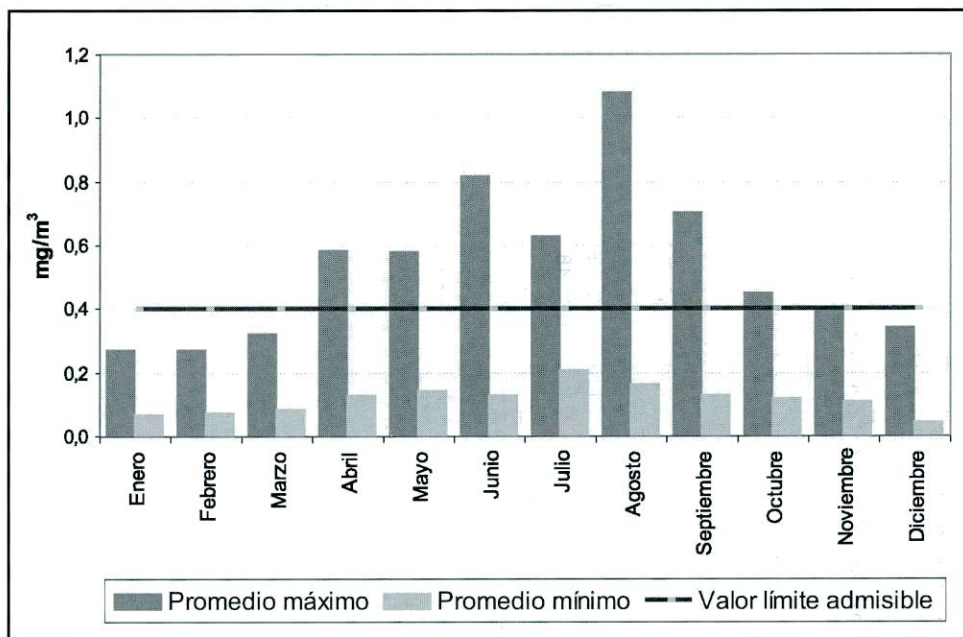
Gráfico 22.4 Promedios máximos y mínimos de óxido de nitrógeno totales. Ciudad de Buenos Aires. Año 2003
