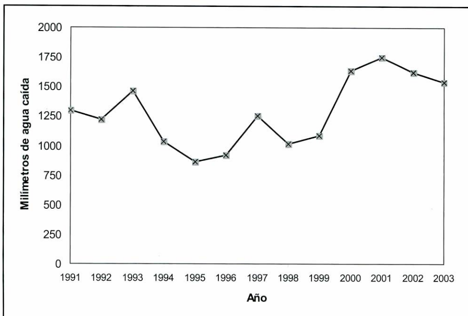
Gráfico 22.3 Precipitaciones. Ciudad de Buenos Aires. Años 1991/2003
