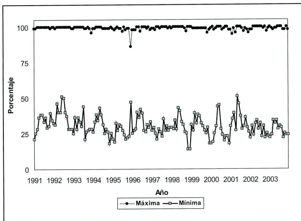
Gráfico 22.2 Porcentaje de los niveles de humedad máximos y mínimos. Ciudad de Buenos Aires. Años 1991/2003
