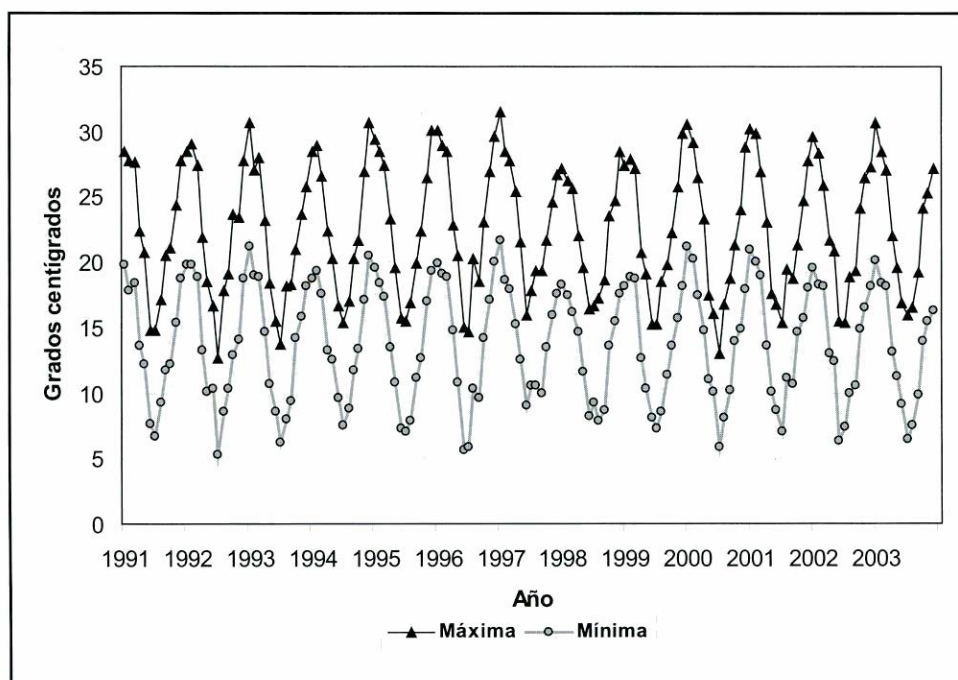
Gráfico 22.1 Temperatura media máxima y mínima. Ciudad de Buenos Aires. Años 1991/2003
